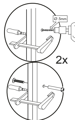
Винт стяжной L32/27
