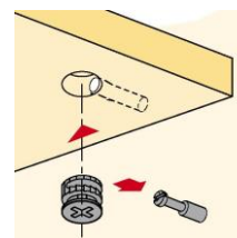
Рис.1 Схема установки стяжки эксцентриковой
