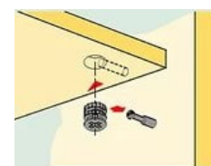
Схема установки Эксцентриковой стяжки
