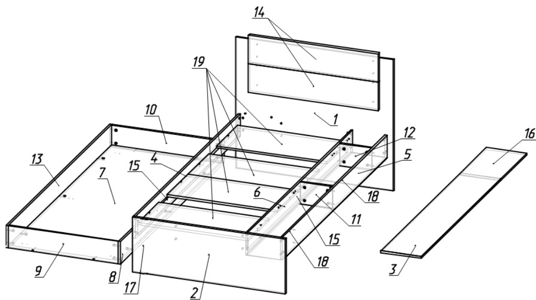
Рис.1 Схема сборки
