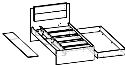
Б – Сборка кровати на правую сторону
